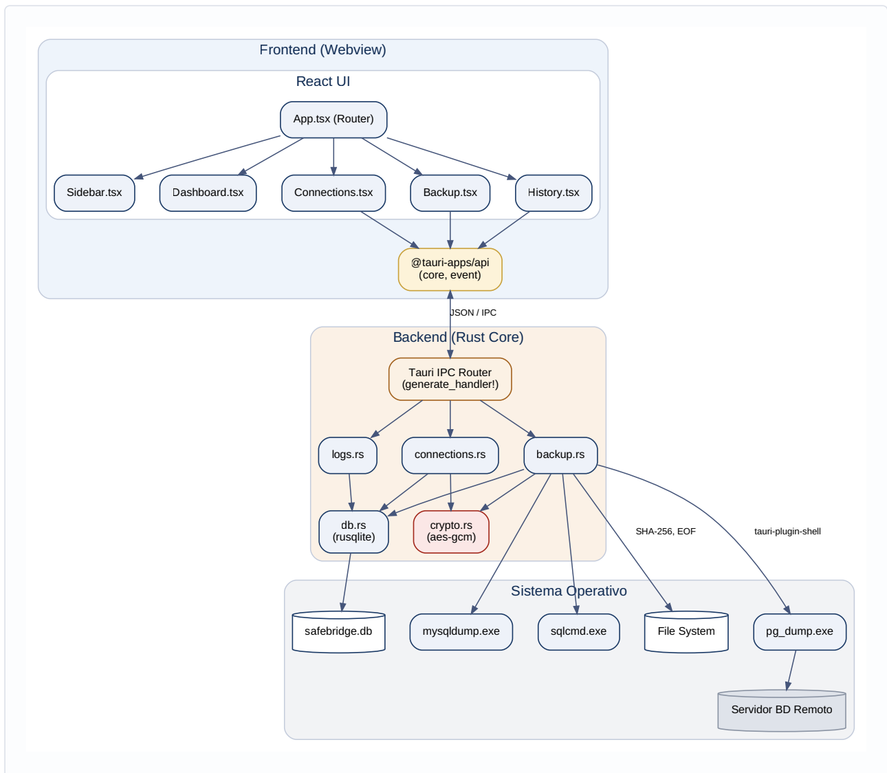
Figura 7 — Diagrama de Componentes del Sistema
