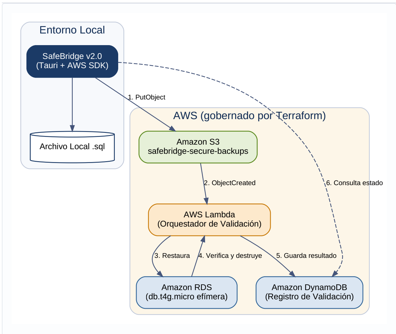
Figura 10 — Infraestructura Teórica en AWS gobernada por Terraform
