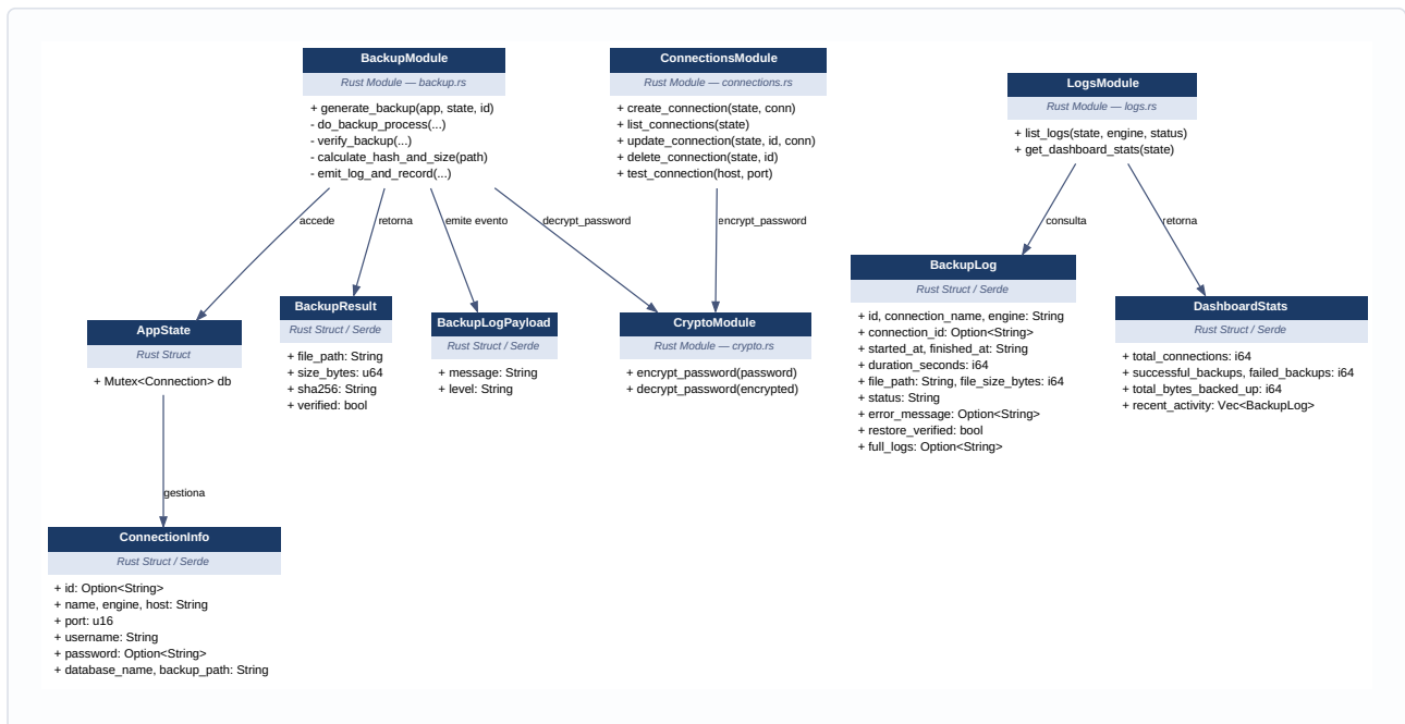
Figura 5 — Diagrama de Clases y Estructuras del Dominio
