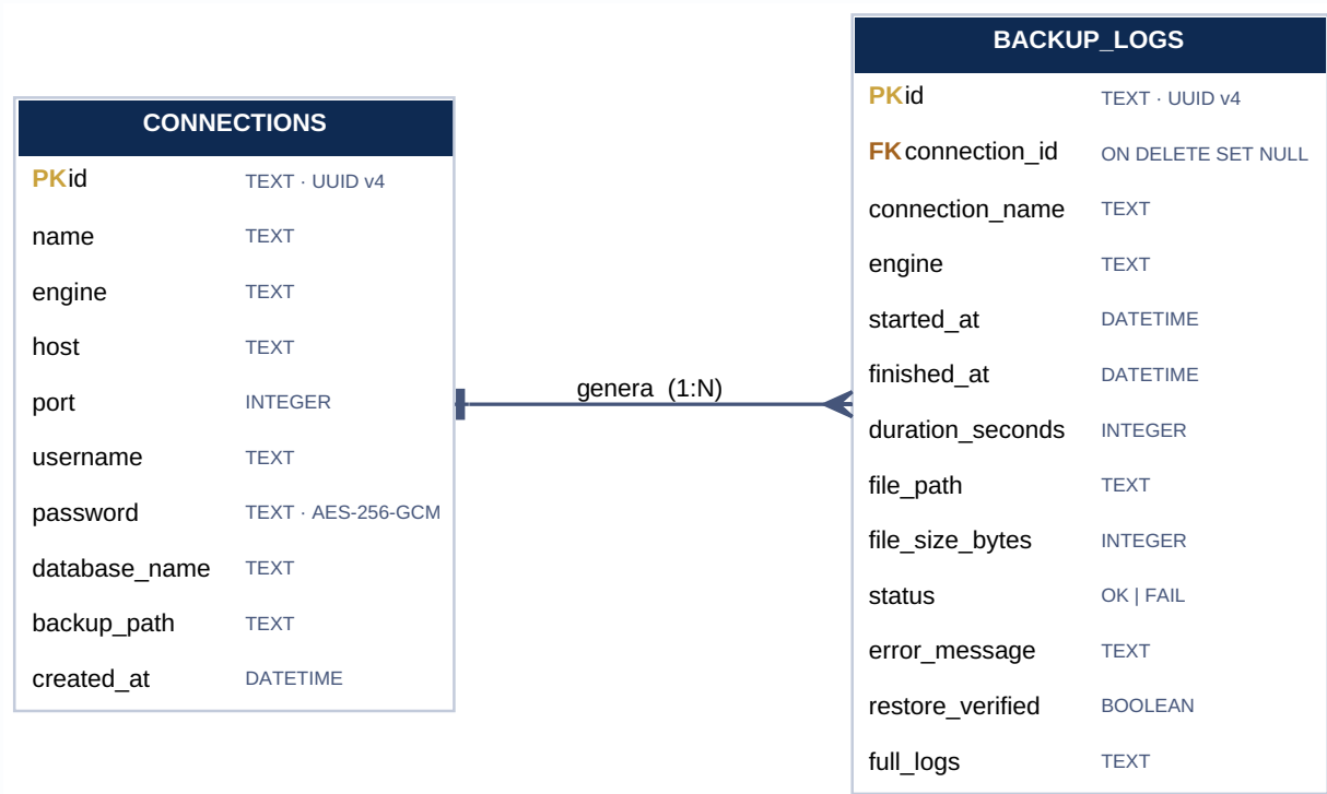
Figura 6 — Diagrama Entidad-Relación de la Base de Datos
