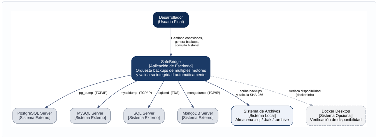
Figura 1.1 — Arquitectura C4 · Nivel 1: Diagrama de Contexto
