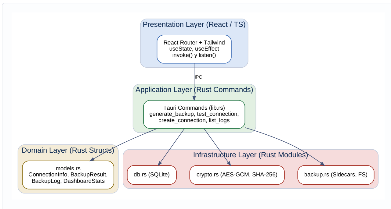
Figura 9 — Diagrama de Arquitectura Clean
