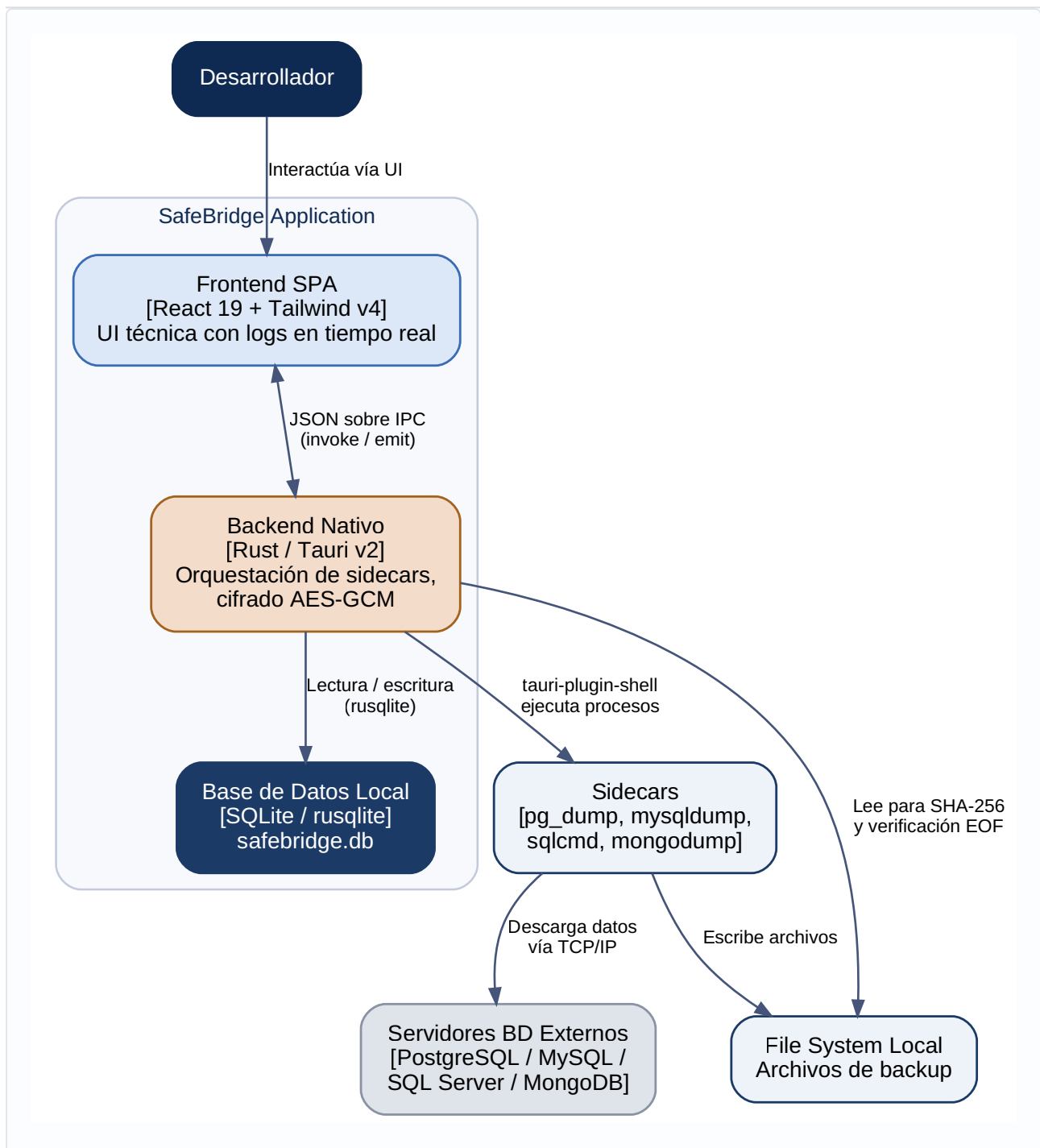
Figura 1.2 — Arquitectura C4 · Nivel 2: Diagrama de Contenedores
