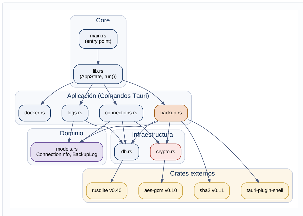
Figura 3.2 — Diagrama de Paquetes del Backend (Rust/Tauri)
