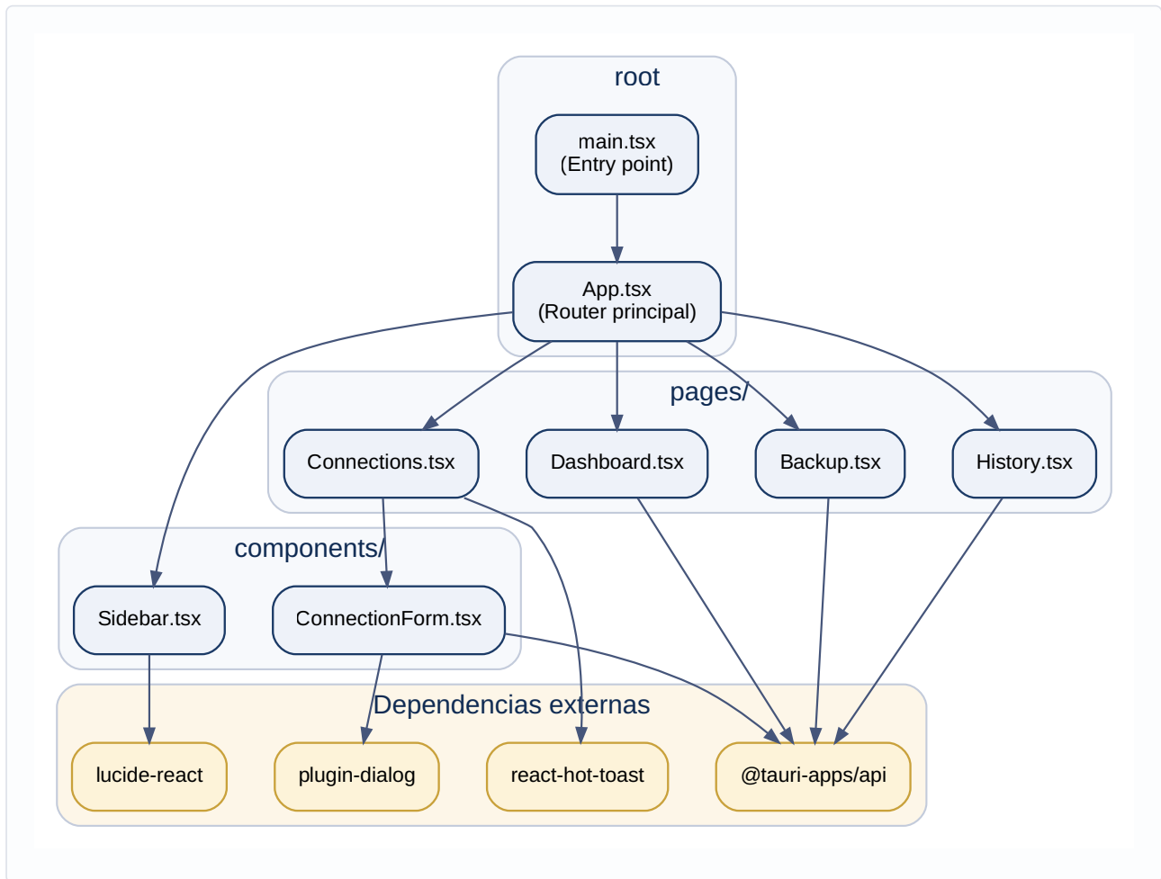
Figura 3.1 — Diagrama de Paquetes del Frontend (React/TypeScript)
