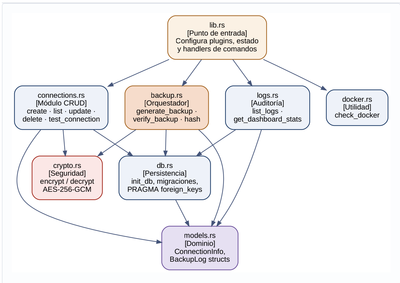
Figura 1.3 — Arquitectura C4 · Nivel 3: Componentes del Backend
