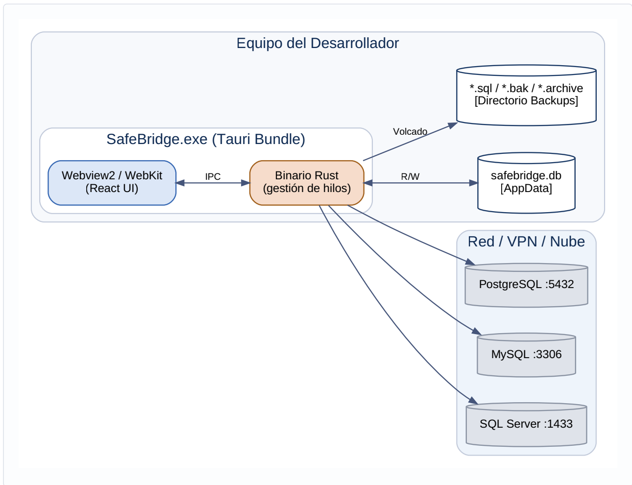
Figura 8 — Diagrama de Despliegue
